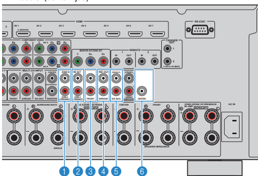
Dit toestel (achterzijde)
