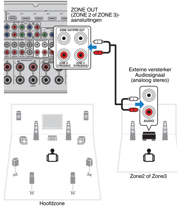
Dit toestel (achterzijde)
