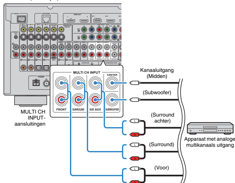
Dit toestel (achterzijde)
