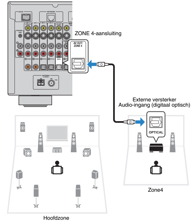
Dit toestel (achterzijde)
