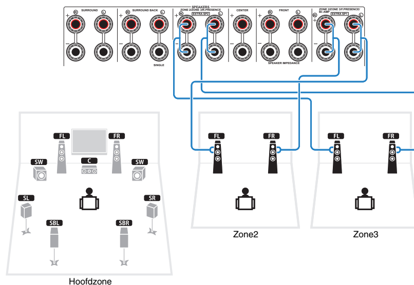
Dit toestel (achterzijde)
